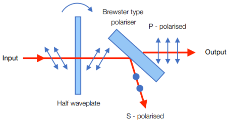
光学设计
